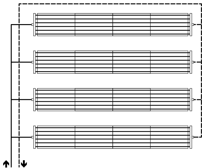
Abb. 14 System Tichelmann mit wechelseitigem Anschluss
