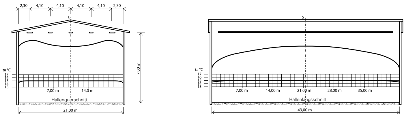
Abb. 12 Strahlungsintensität und Raumtemperatur bei Verwendung von leistungstärkeren Paneelen an der Randzone
