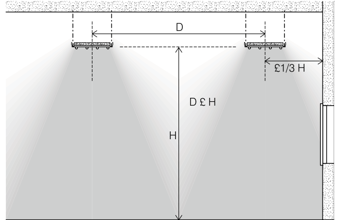
Abb.10 Paneelabstand zueinander
