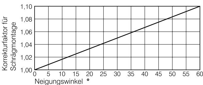
Abb.9 Korrekturfaktor für Schrägmontage
