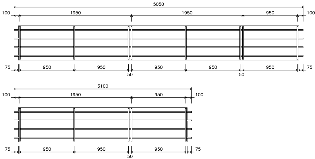
Abb.2 Längenmaße und Aufhängeabstände der Sondermodule 3 und 5 m (mm)
