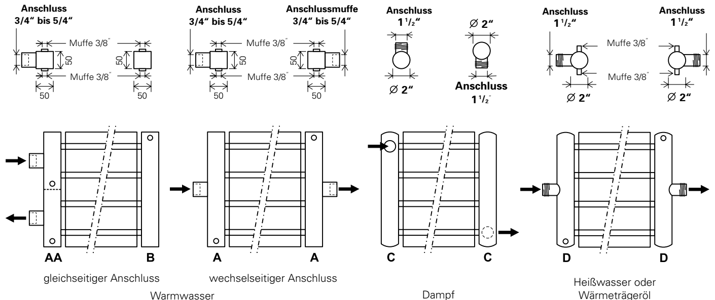
Abb.3 Sammlerköpfe - Ausführung AA,B,A,C,D (mm)
